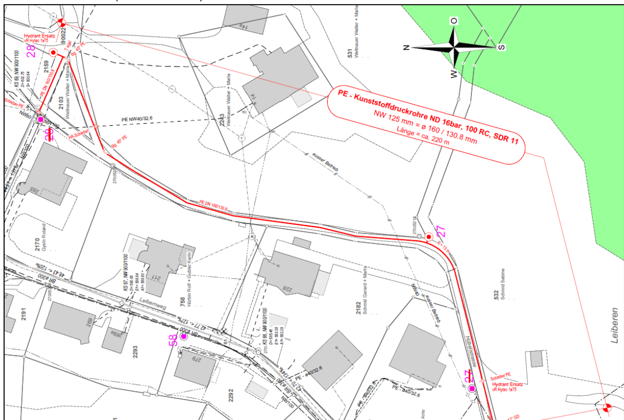
Ausschnitt aus dem GWP (nicht massstäblich)
